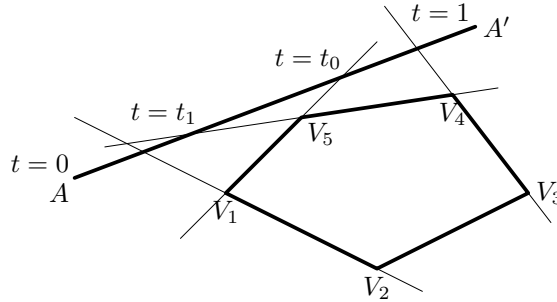
OBR. 2. Hľadanie prieniku úsečky a konvexného mnohouholníka.
