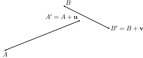
OBR. 1. Hľadanie prieniku dvoch úsečiek. Bázy \mathbf{u}, B - A a \mathbf{u}, B' - A sú opačne orientované, ale bázy \mathbf{v}, A - B a \mathbf{v}, A' - B sú zhodne orientované, a preto úsečky nemajú spoločný bod.
