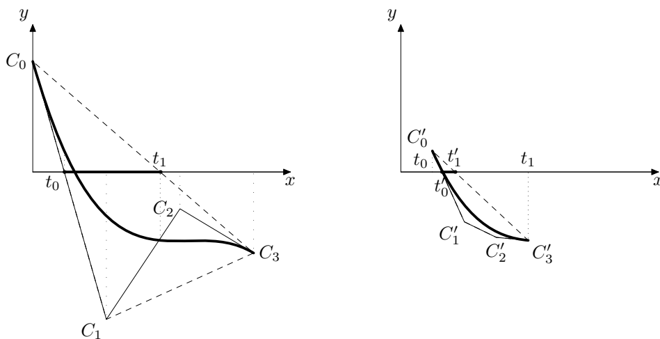
OBR. 3. Hľadanie koneňa polynomickej rovnice Beziérovým orezávaním.
