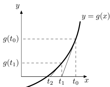
OBR. 4. Hľadanie koreňa rovnice y = g(x) Newtonovou metódou.
