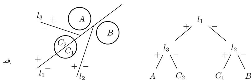
OBR. 3. Usporiadanie scény do BSP stromu
