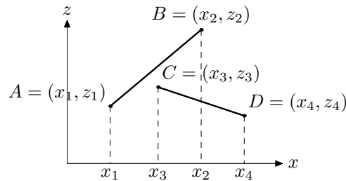
OBR. 2. Intervaly na zametacej priamke
